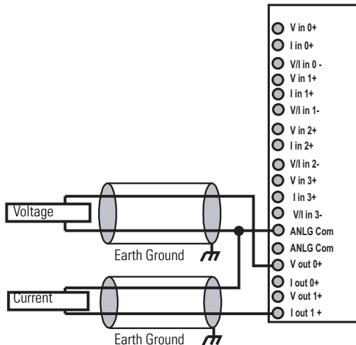
1769-IF4XOF2 Outputs
