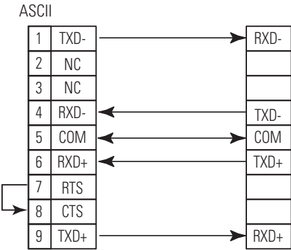
RS-485 Wiring
