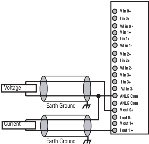
1769-IF4FXOF2F Outputs
